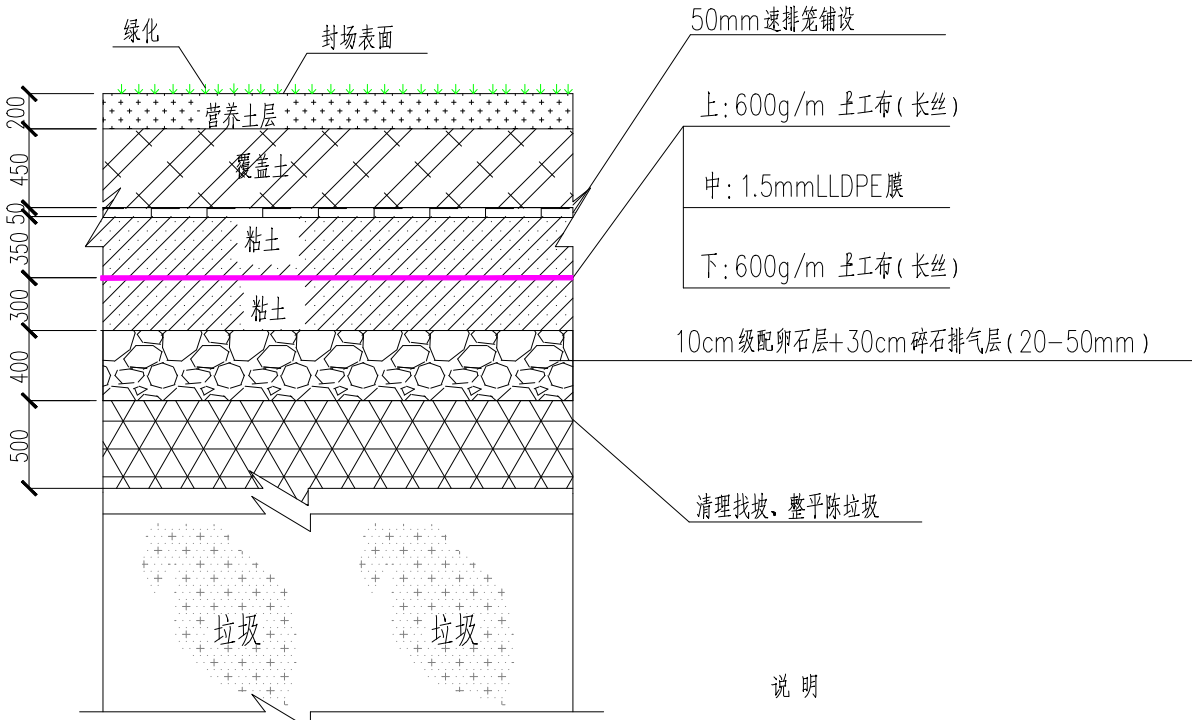
填埋场封场覆盖体结构
